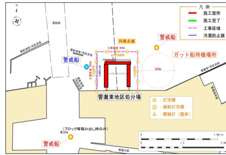
図-5 工事作業警戒船配置図
