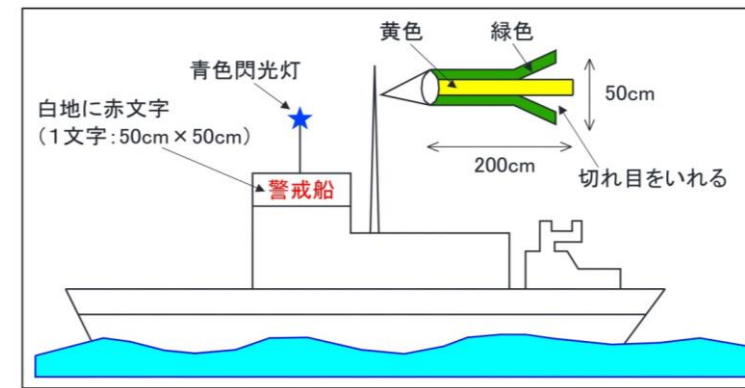
図-4 工事作業警戒船イメージ図
