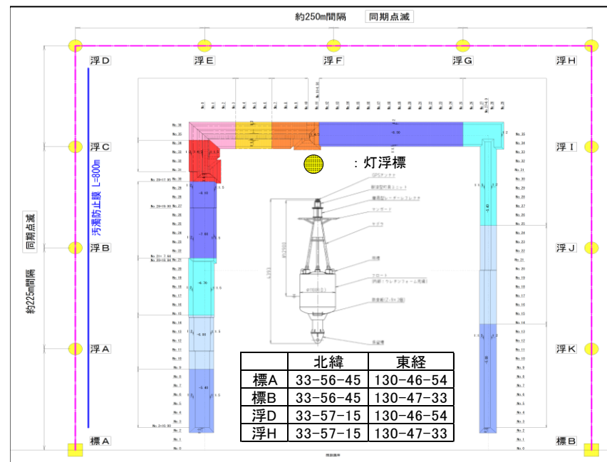
図-2 護岸築造工事平面図
