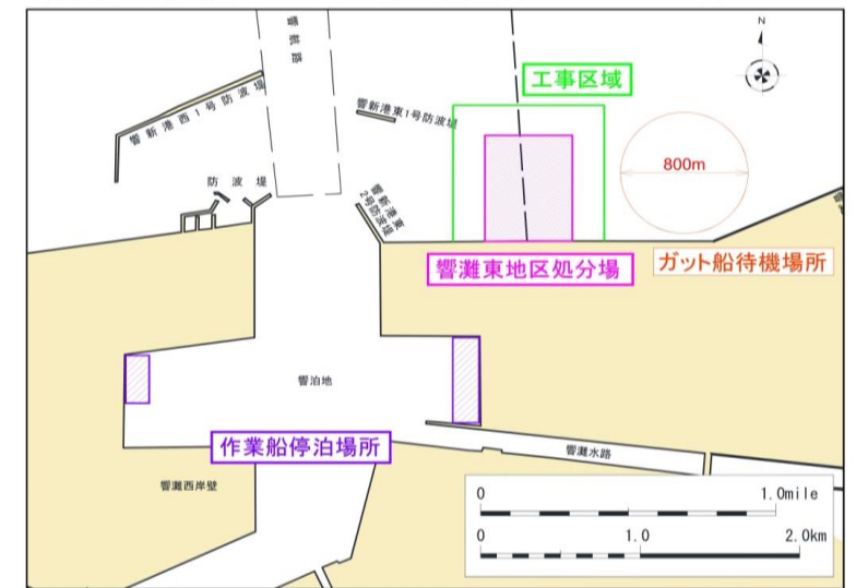
図-6 作業船待機場所図
