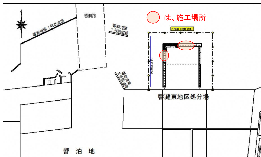
図-1 護岸築造工事位置図
