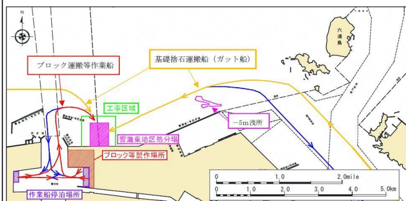
図-3 作業船運航経路図
