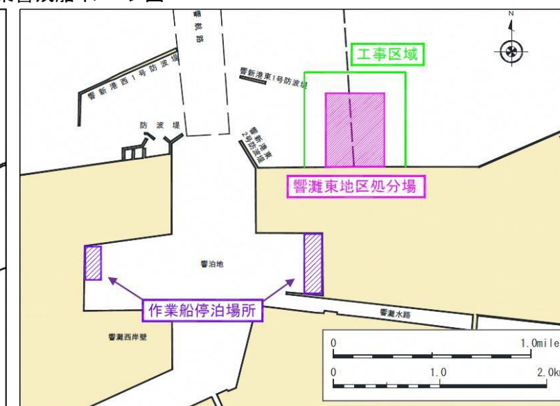
図-6 作業船停泊場所図
