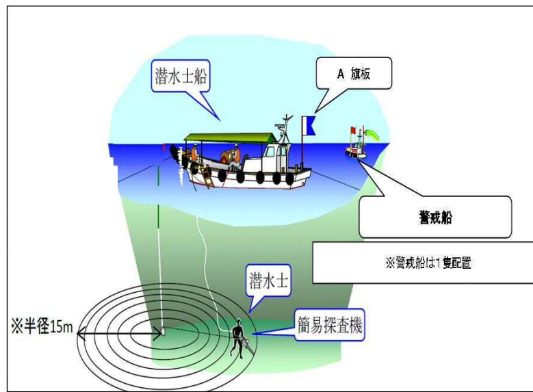
図2 潜水探査概念図
