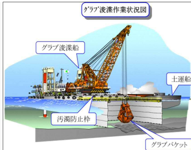
図3 グラブ浚渫概念図
