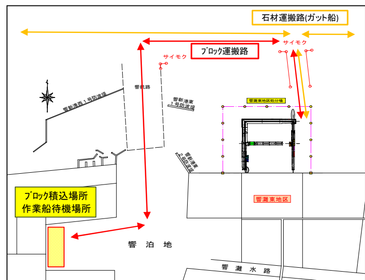
図-3 運搬経路図
