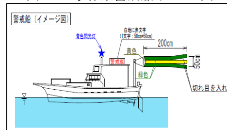
図-4 工事作業警戒船イメージ図
