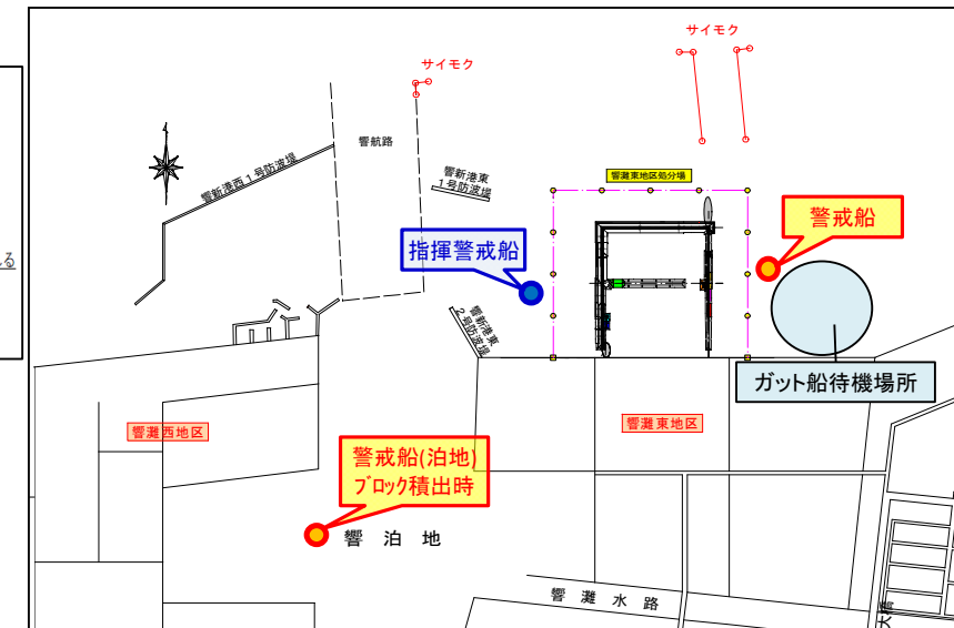
図-5 工事作業警戒船配置図
