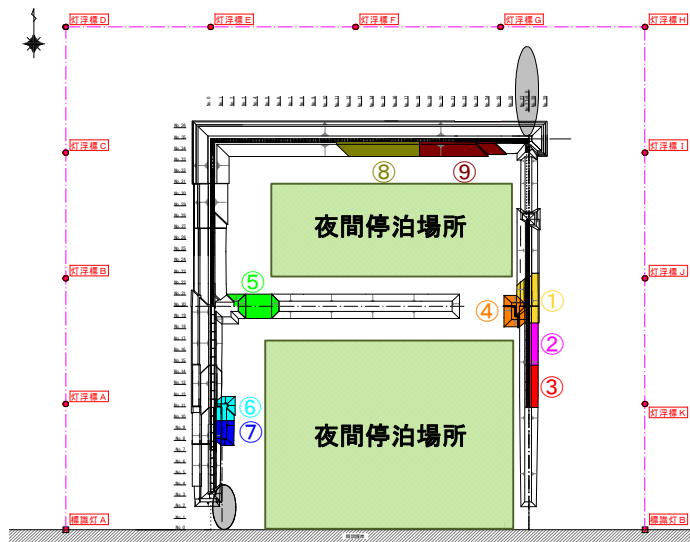
図-1 護岸築造工事位置図
