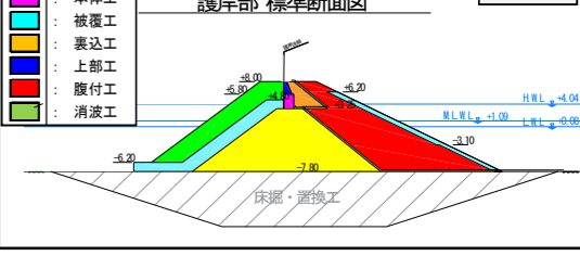
図-5. 護岸部標準断面図
